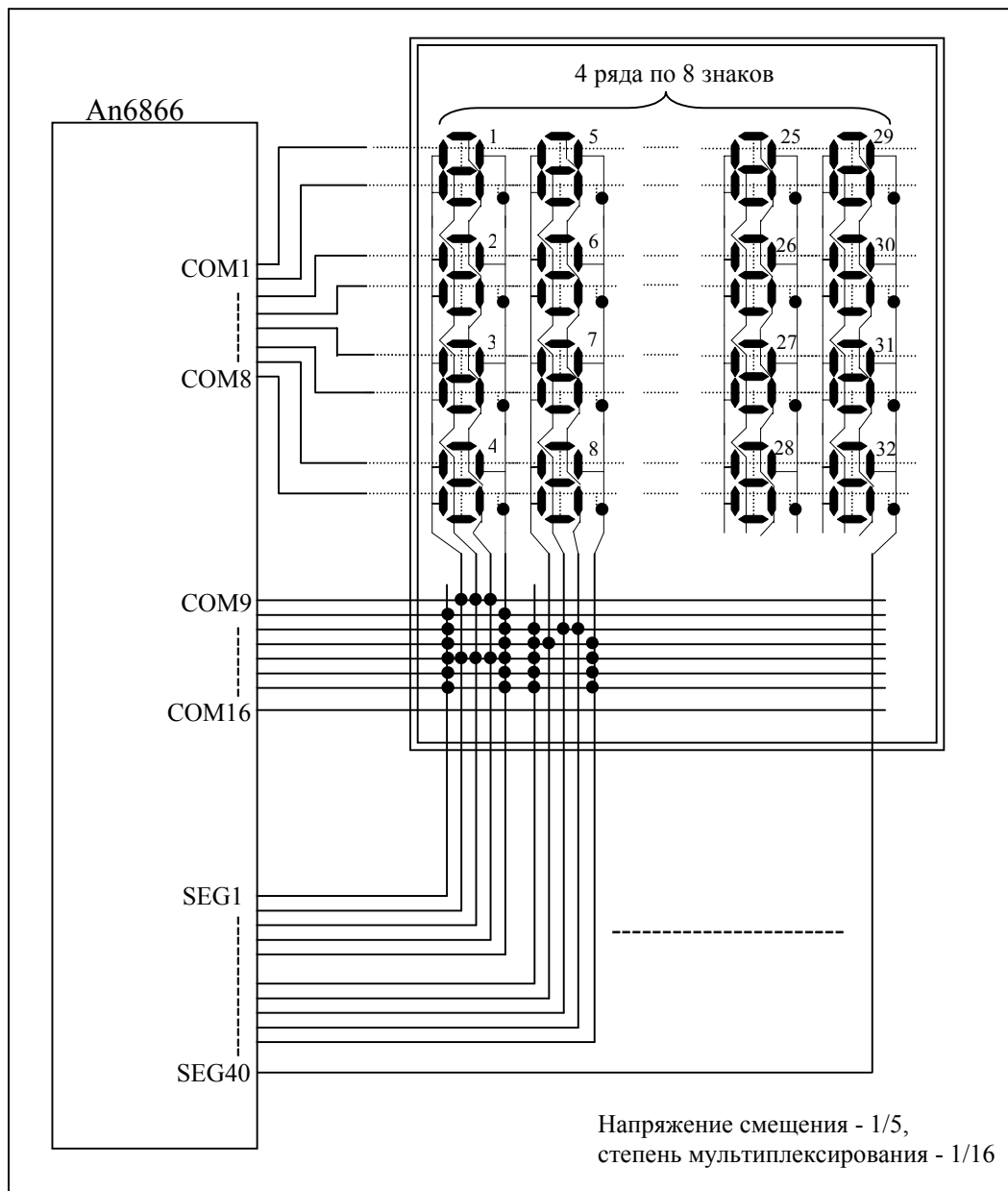
Рис. 29. Схема отображения 32 7-сегментных знаков и 8 символьной текстовой строки
