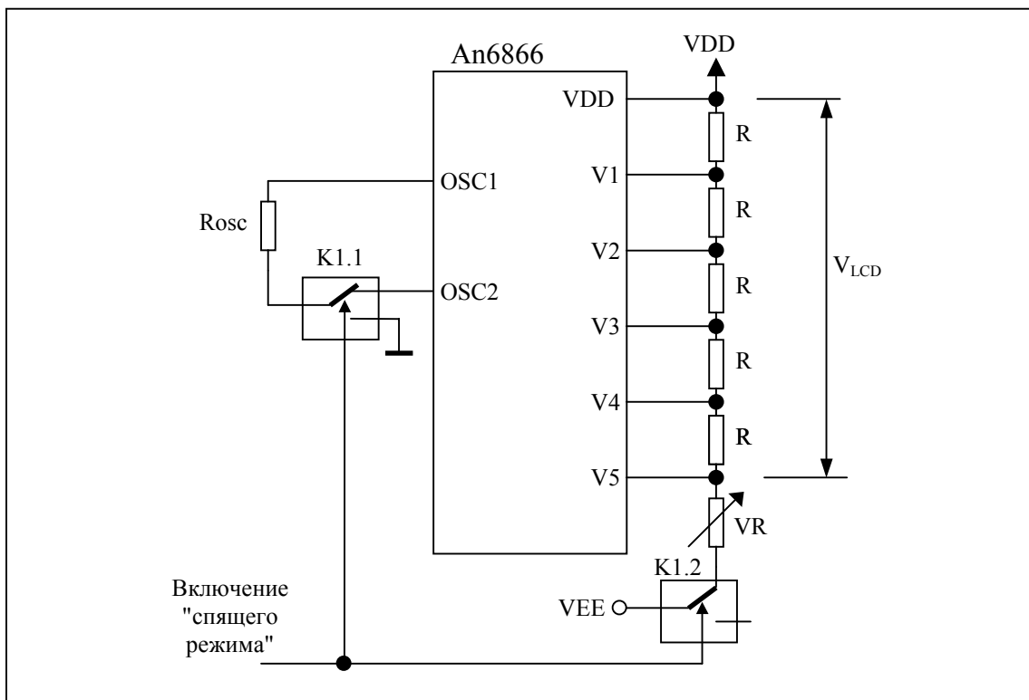
Рис. 27. Организация "спящего" режима
