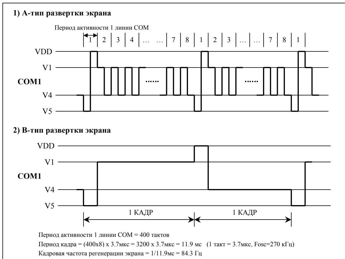
Рис. 16. Временная диаграмма сигналов развертки экрана для степени мультиплексирования 1/8
